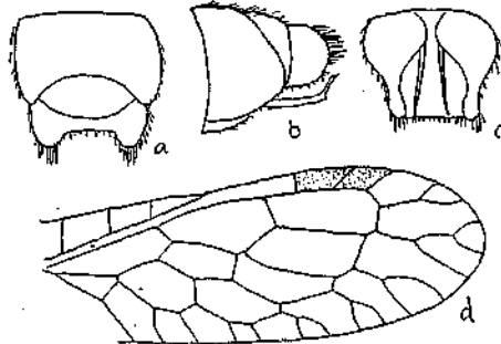
Fig. 9. Raphidilla puella ♂ Nav.
