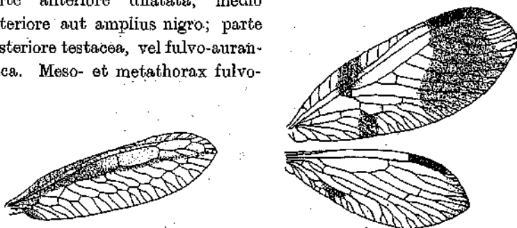
Fig. 7. Climaciella Duckei Nav. Fig. 8. Symphrasis thaumasta ♂ Nav. Vorderflügel, \times 2\frac{1}{2} (Mus. von Bern). Flügel, \times 5 . (Mus. von Bern.)
