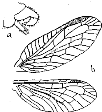
Fig. 12. Sialis fumosa ♂ Nav. a) Hinterleibsende von der Seite. b) Die Flügel, × 4. (Coll. m.)
